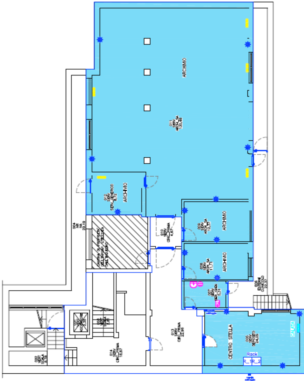
Agenzia delle Entrate DP Gorizia PIANTA PIANO INTERRATO
