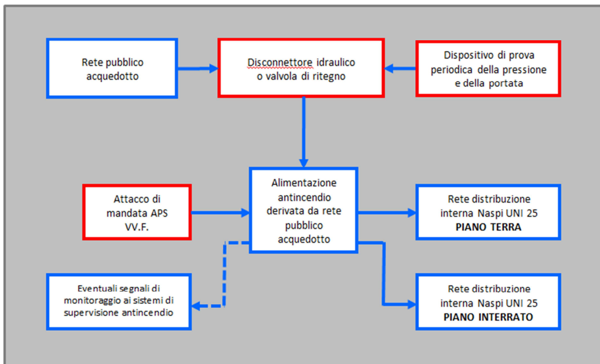
Tipico esempio di impianto di rete idranti:
