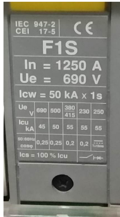
Interruttore a carrello a servizio del sistema di commutazione rete normale/preferenziale – dati tecnici
