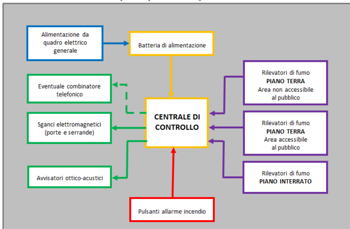
Esempio di impianto di rivelazione allarme
