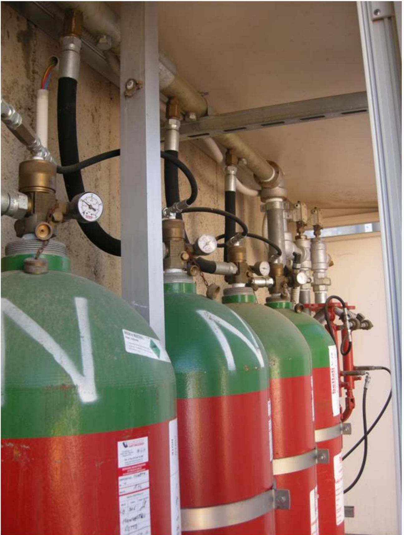
Foto n. 3 – gruppo bombole
